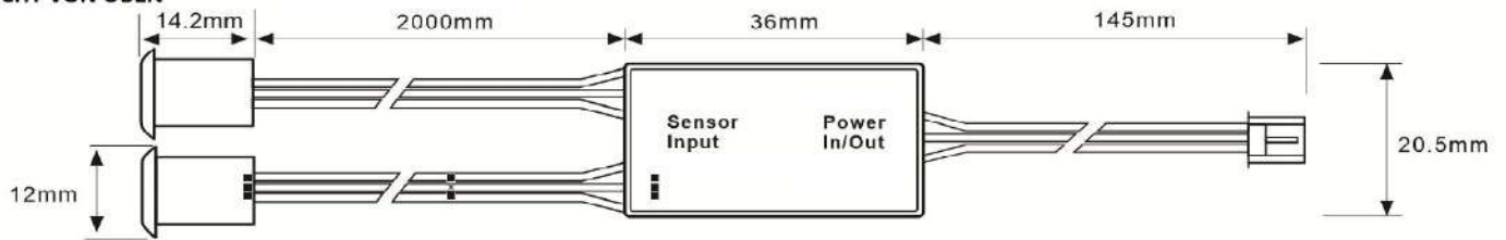
SEITENANSICHT
